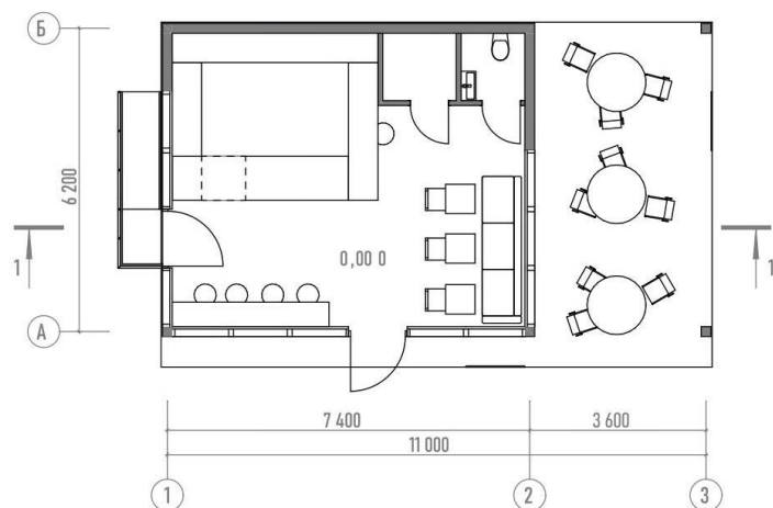
Схема плана
