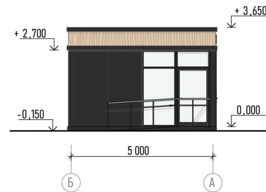
Фасад Б-А
