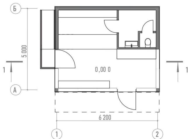
Схема плана
