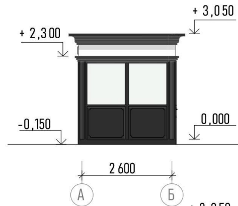
Фасад А-Б
