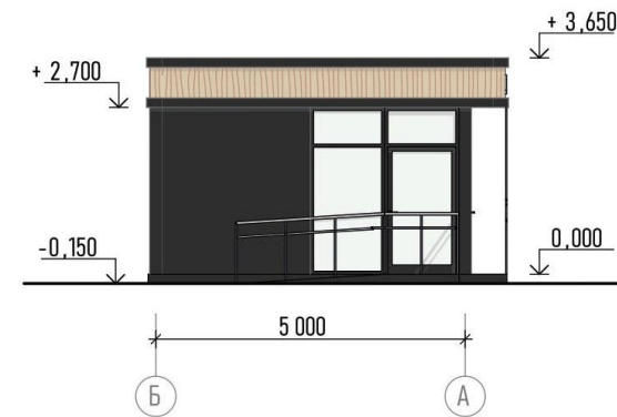
Фасад Б-А
