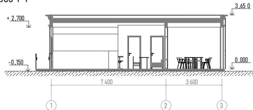
Разрез 1-1
