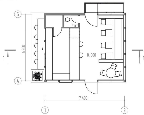
Схема плана
