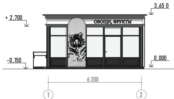
Фасад 1-2
