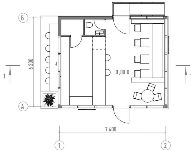
Схема плана
