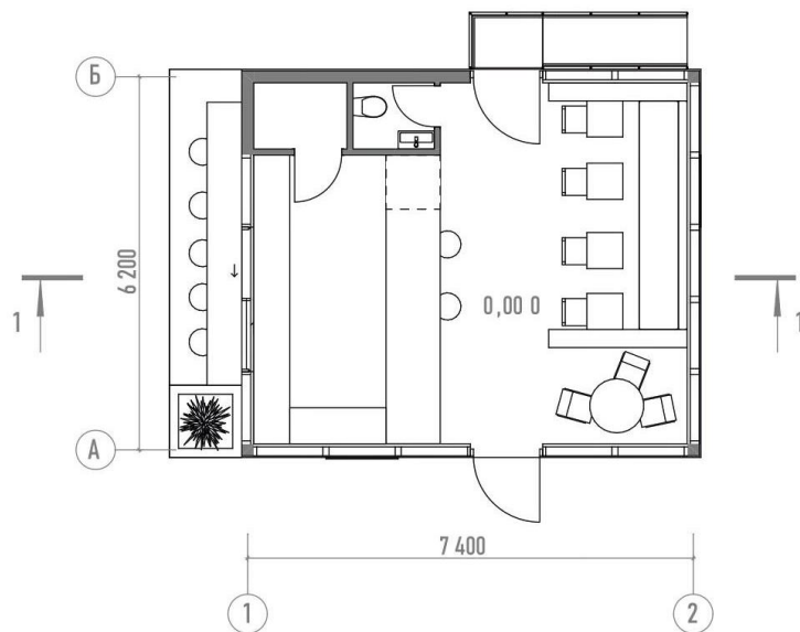
Схема плана
