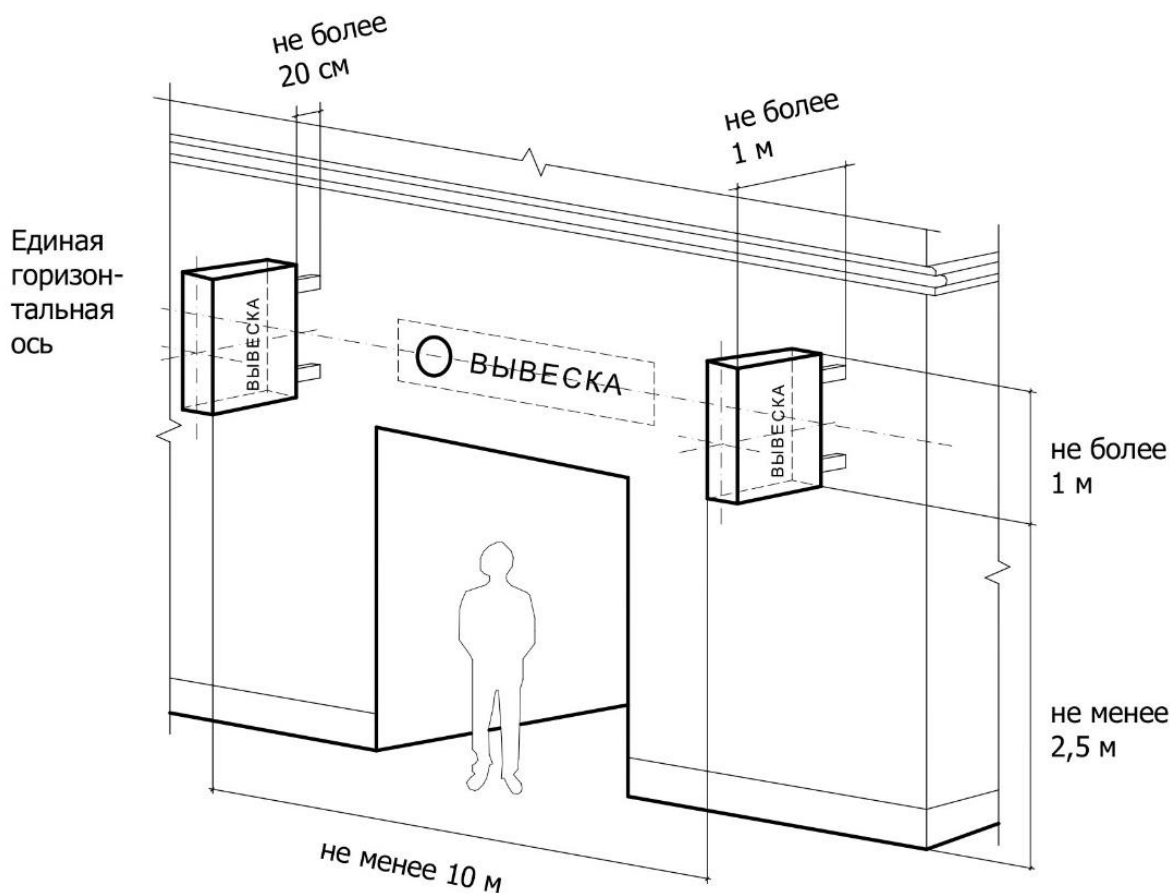
Рисунок 1 – Размещение панелей-кронштейнов на фасаде здания
