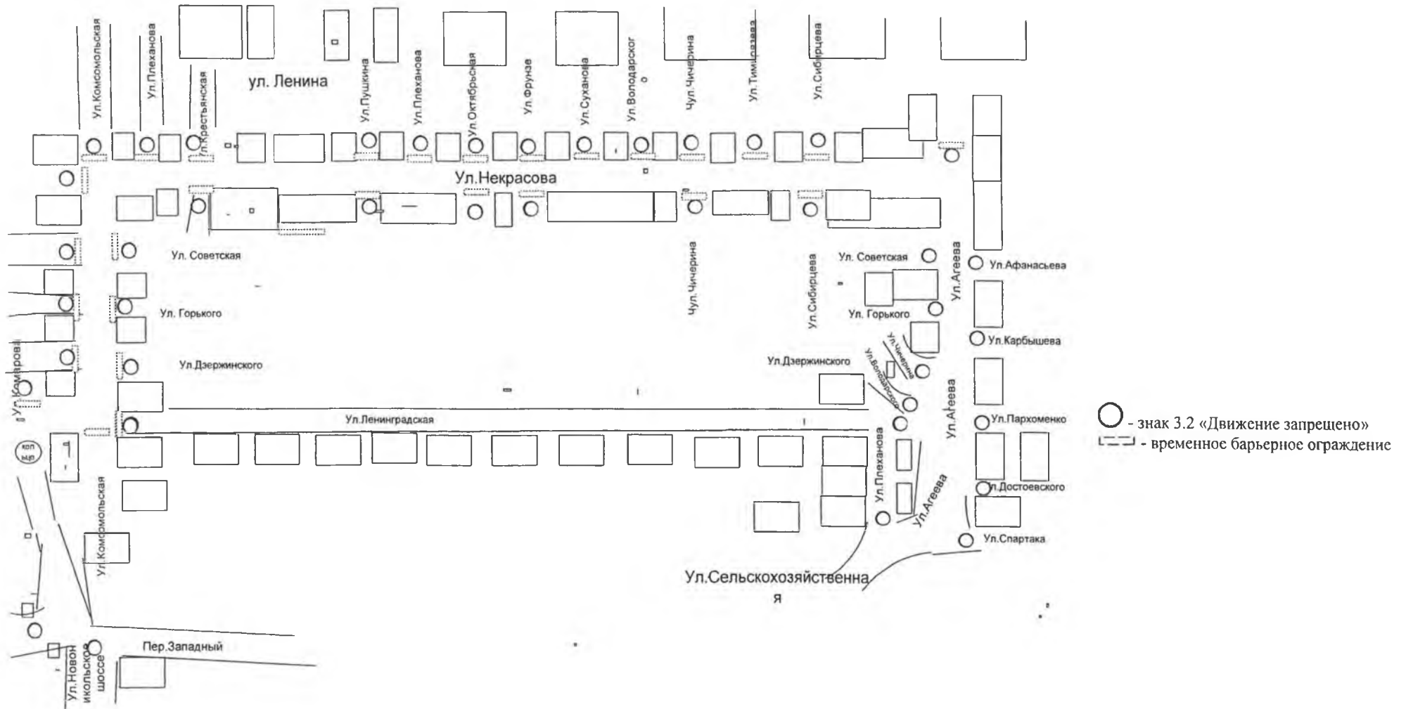
Схема организации перекрытия дорожного движения и маршрутов (лист – 1)
